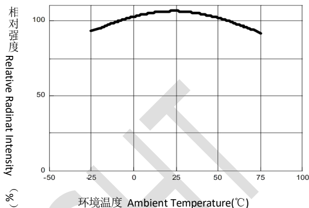
输出特性
