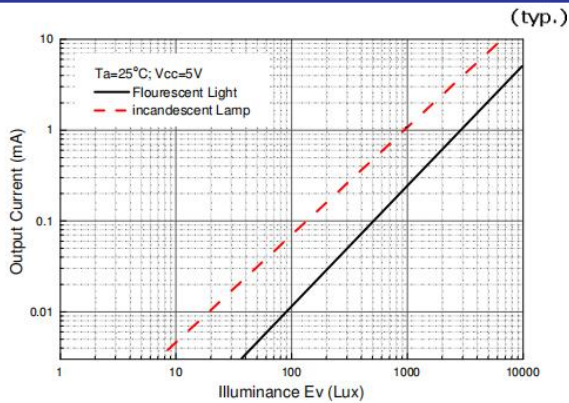
电流与照度的关系 Light Current vs. Illuminance
