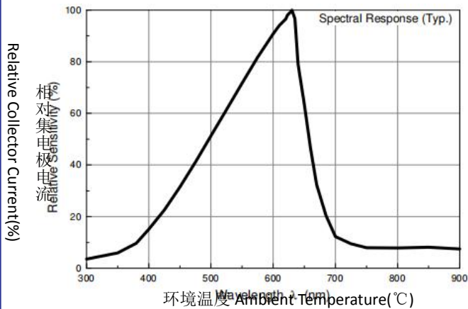
光谱响应 Spectral Response
