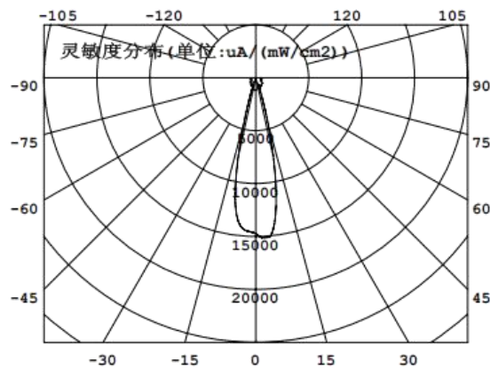
灵敏度分布数据: (角度°, uA/(mW/cm2)) C0-180
