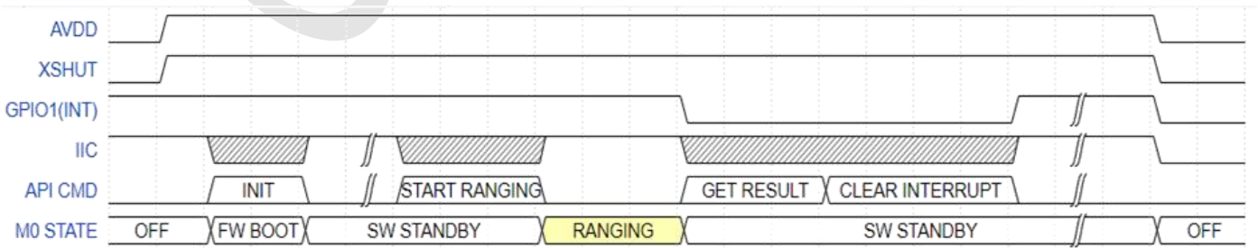
图 6 上电启动时序图
