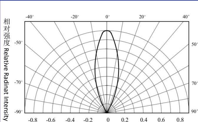
相对辐射强度与角位移的关系 Relative Radiant Intensity vs. Angular Displacement
